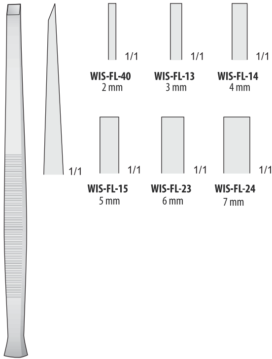
PARTSCH WIS-FL-13/WIS-FL-40 140 mm
