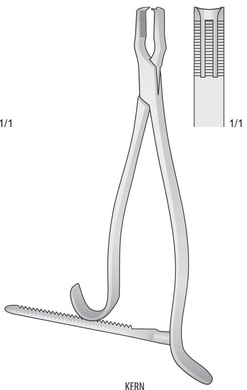
KERN WIS-FO-110 170 mm WIS-FO-112 220 mm
